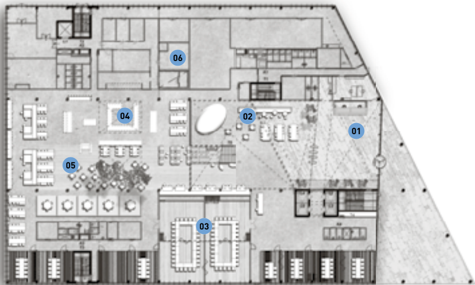
BEGANE GROND
